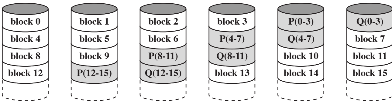
(d) RAID 6 (dual redundancy)
